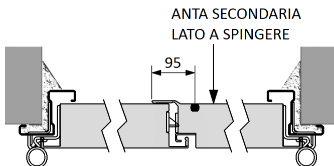
SEZIONE ORIZZONTALE
