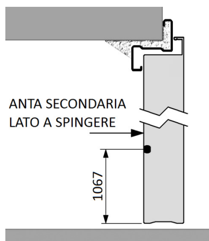
SEZIONE VERTICALE
